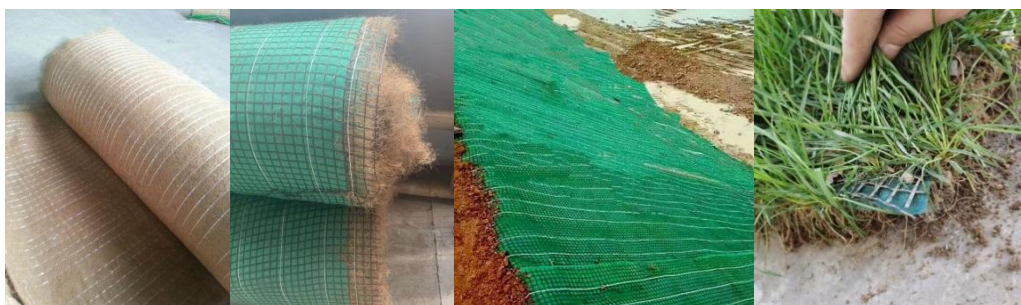
图 C.6 植物纤维毯（垫）防护示例
